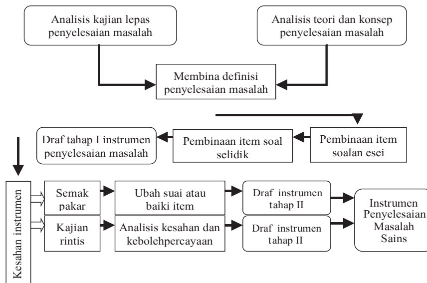
RAJAH 1. Carta aliran Sistematik Metodologi Pembangunan Instrumen Penyelesaian Masalah Sains
